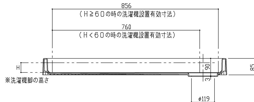
断面A-A
